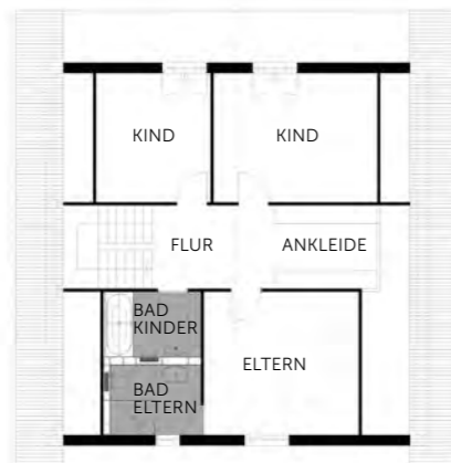
OBERGESCHOSS
